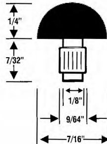
M-827-D Knurled Stud
